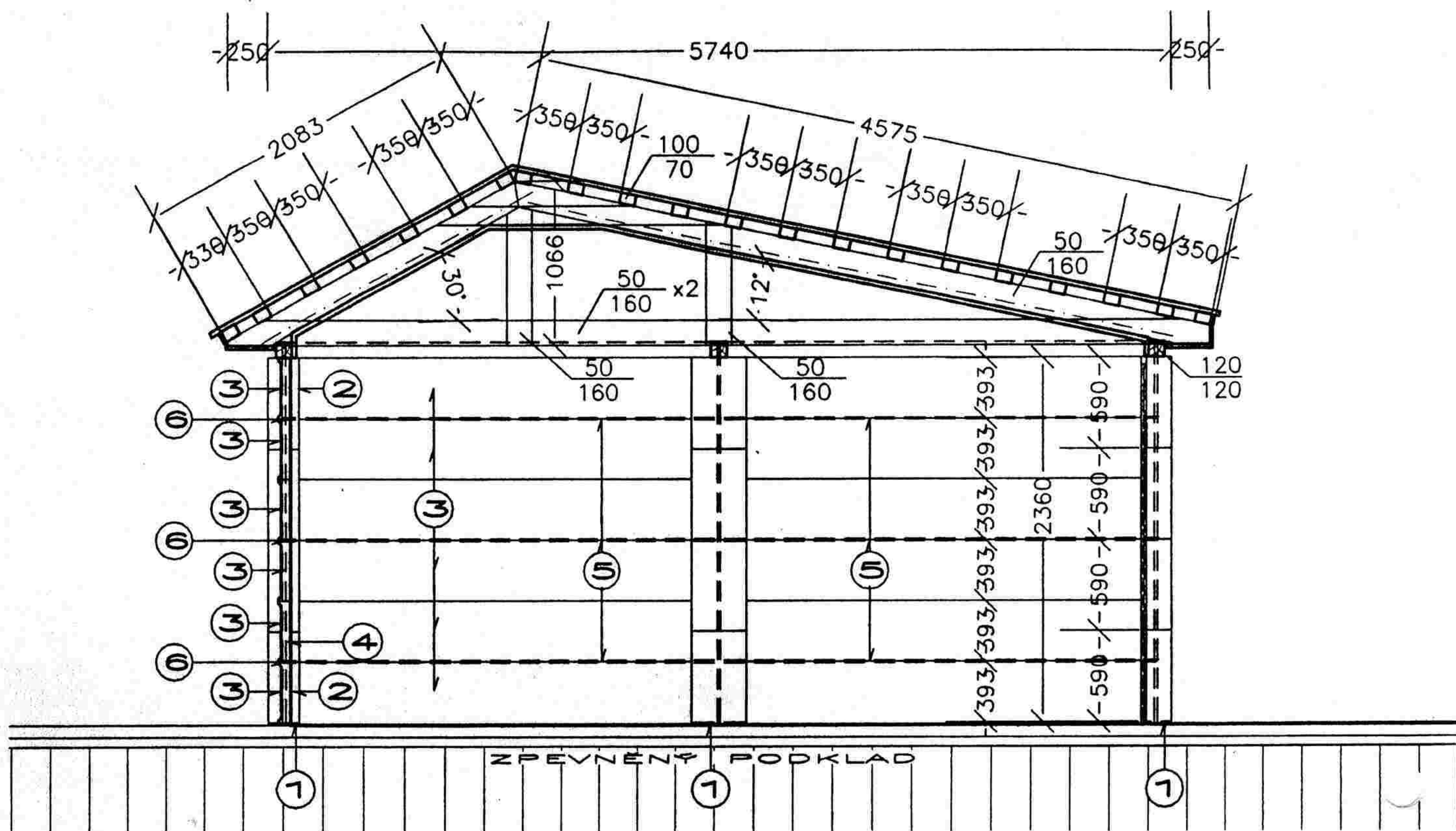
PODELNÝ ŘEZ : 2-2'
