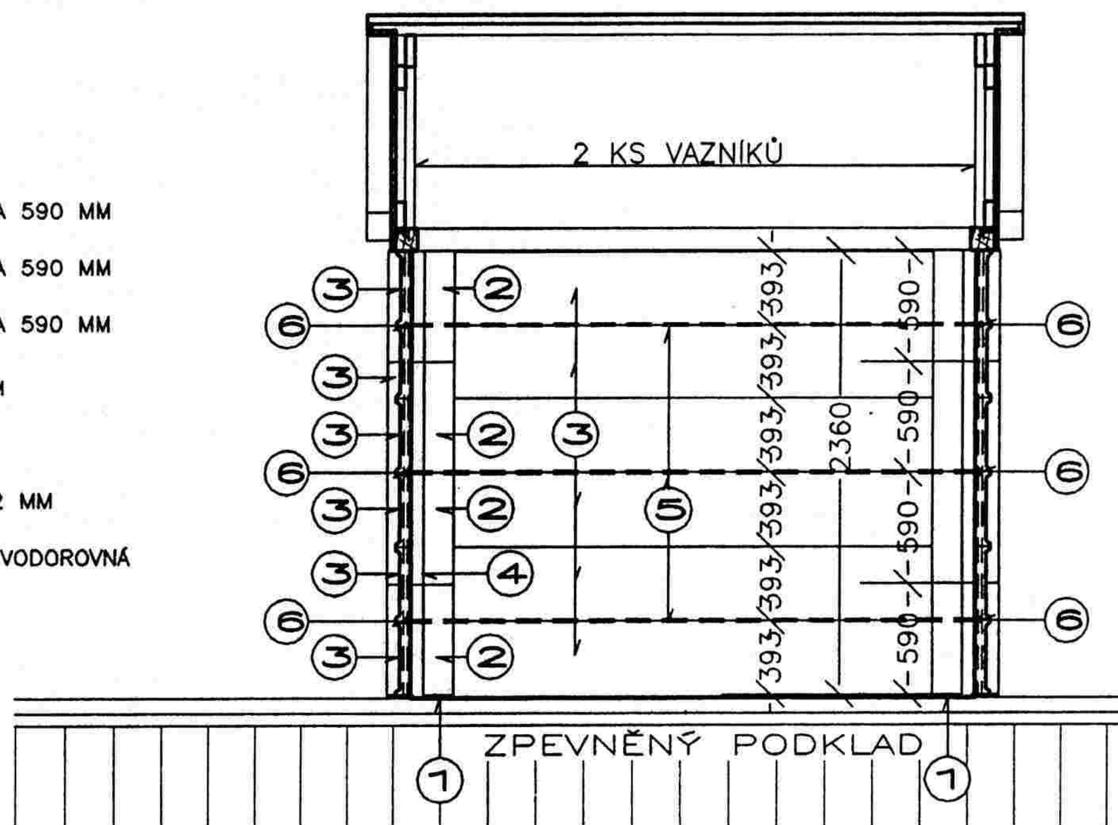
PŘÍČNÝ ŘEZ : 1-1'
